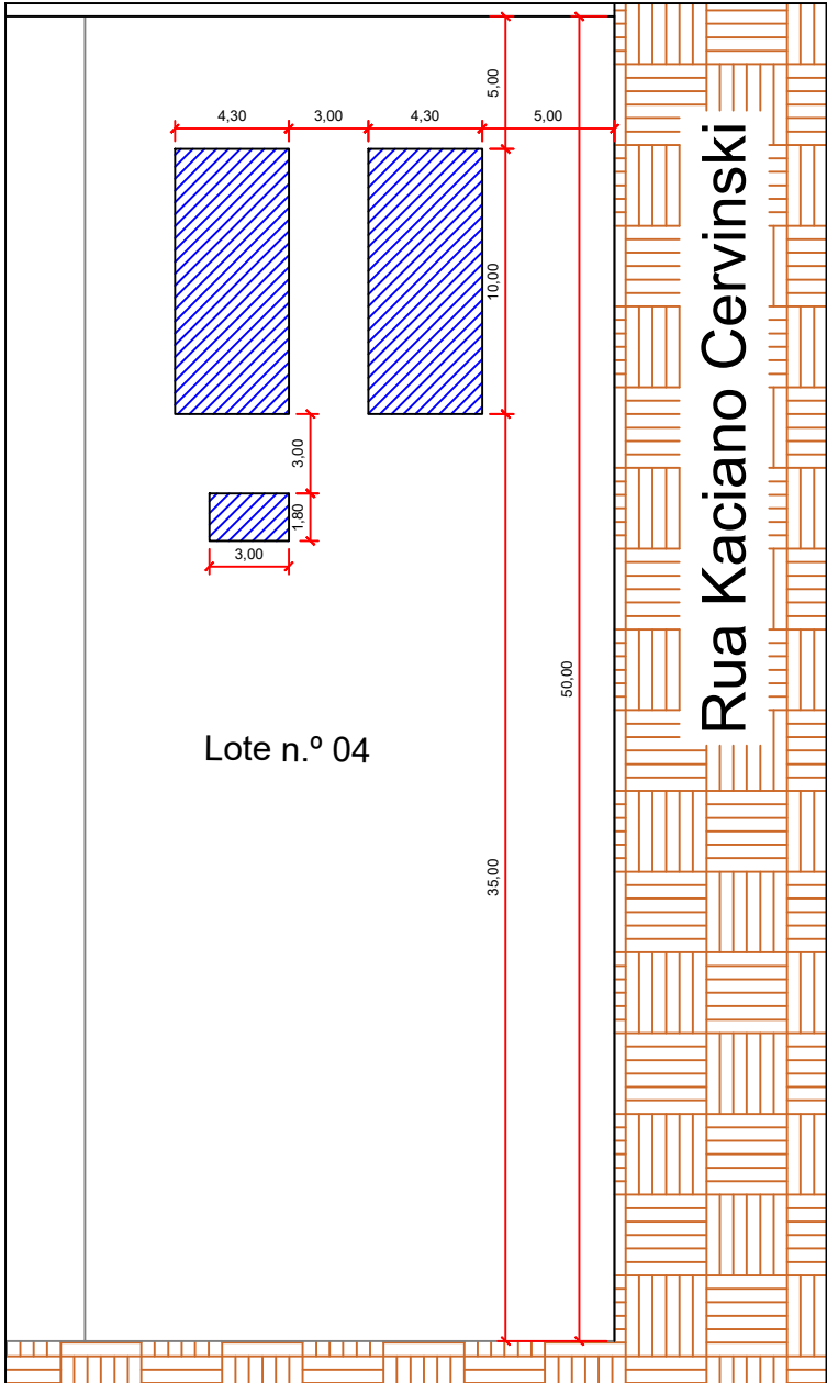
Planta de locação S/ESC
