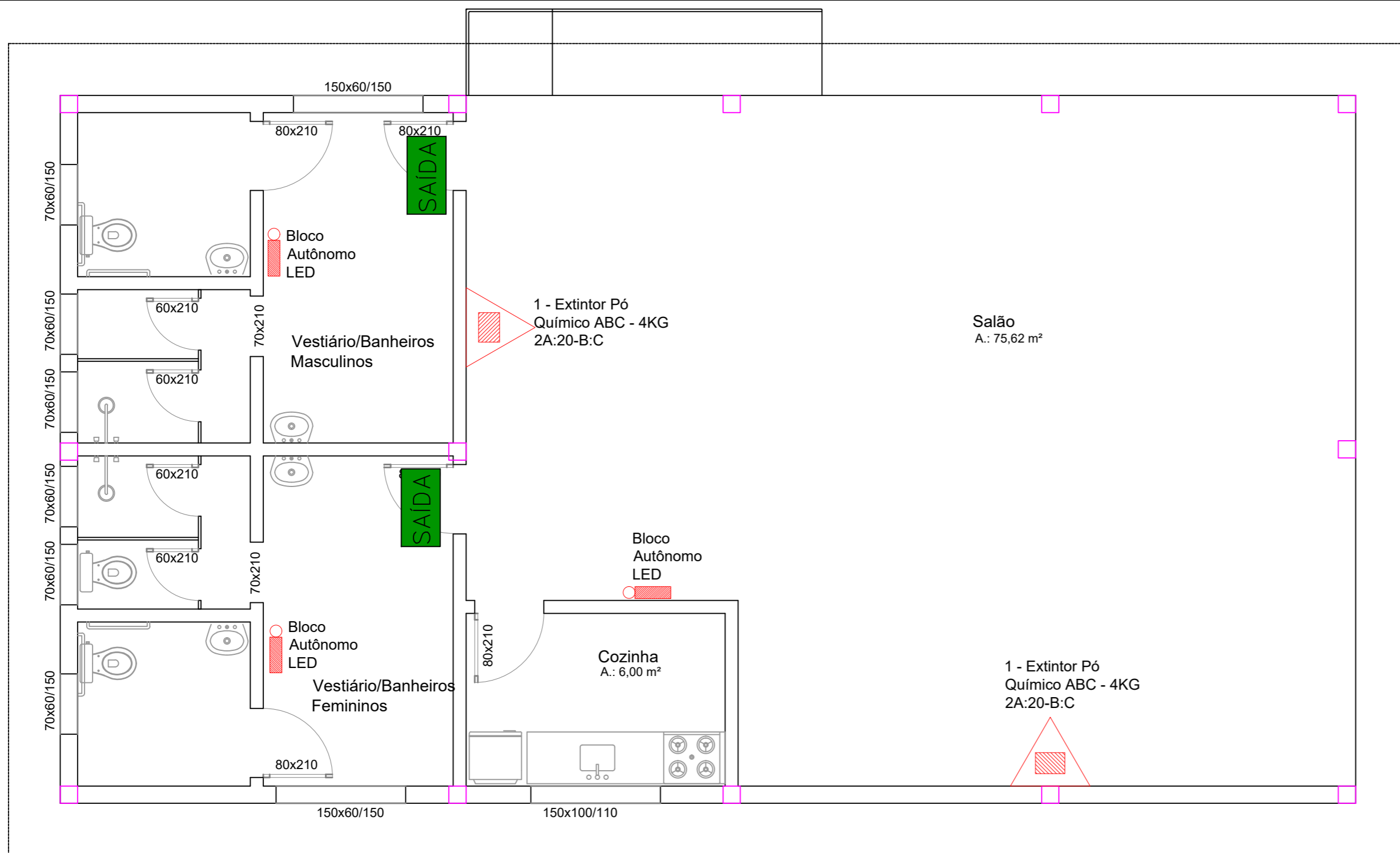
Planta Baixa Sede ESC 1:50
