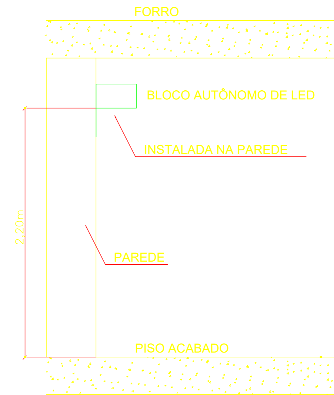
Detalhe execução blocos autônomos S/ESC.
