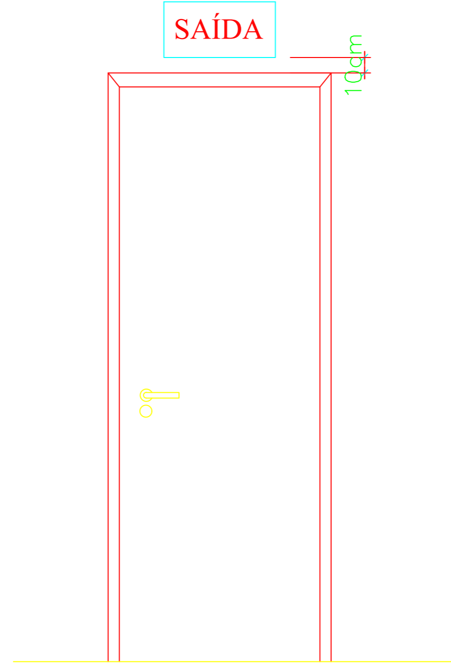
Detalhe execução sinalização S/ESC.
