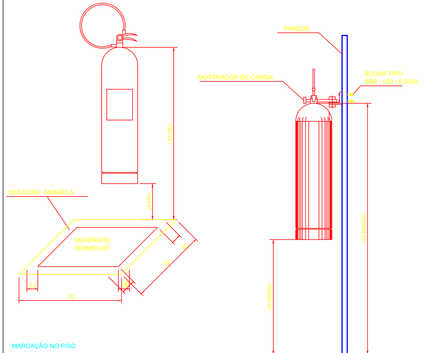
Detalhe execução extintores S/ESC.
