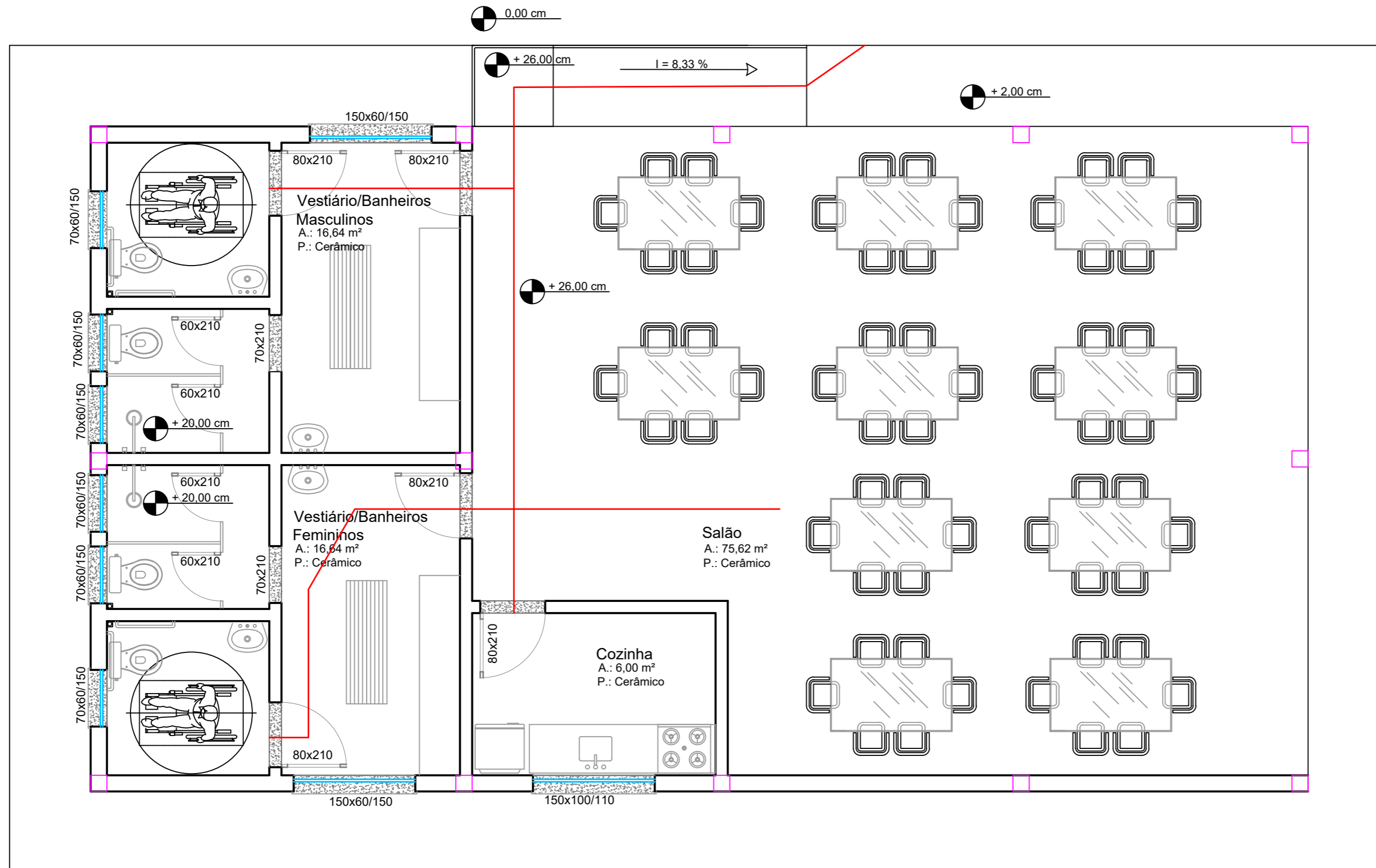
Planta Baixa com rota acessível ESC 1:50
